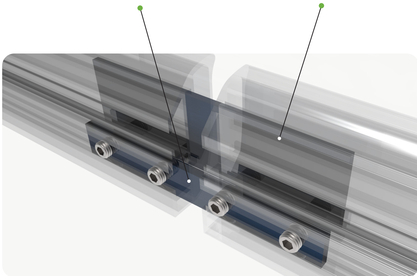
AERO A - Méplat de jonction R4T
